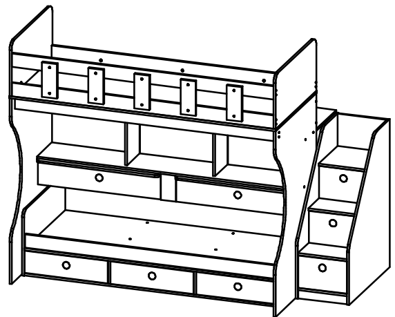
Apm.0710.M1 2386x1255x1800 мм.
