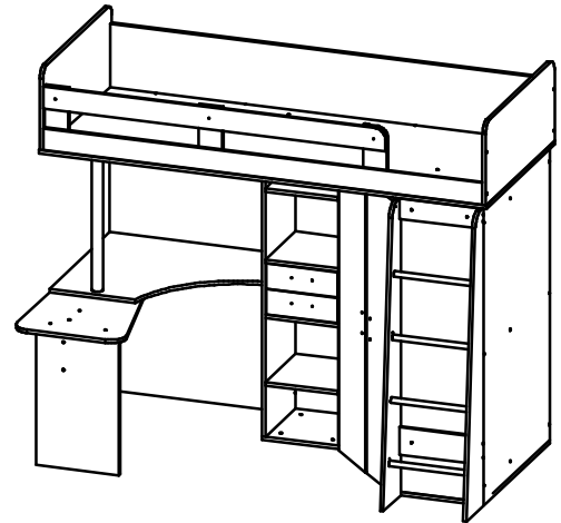
Apm.0705.M1 2068x1281x1790 мм.
